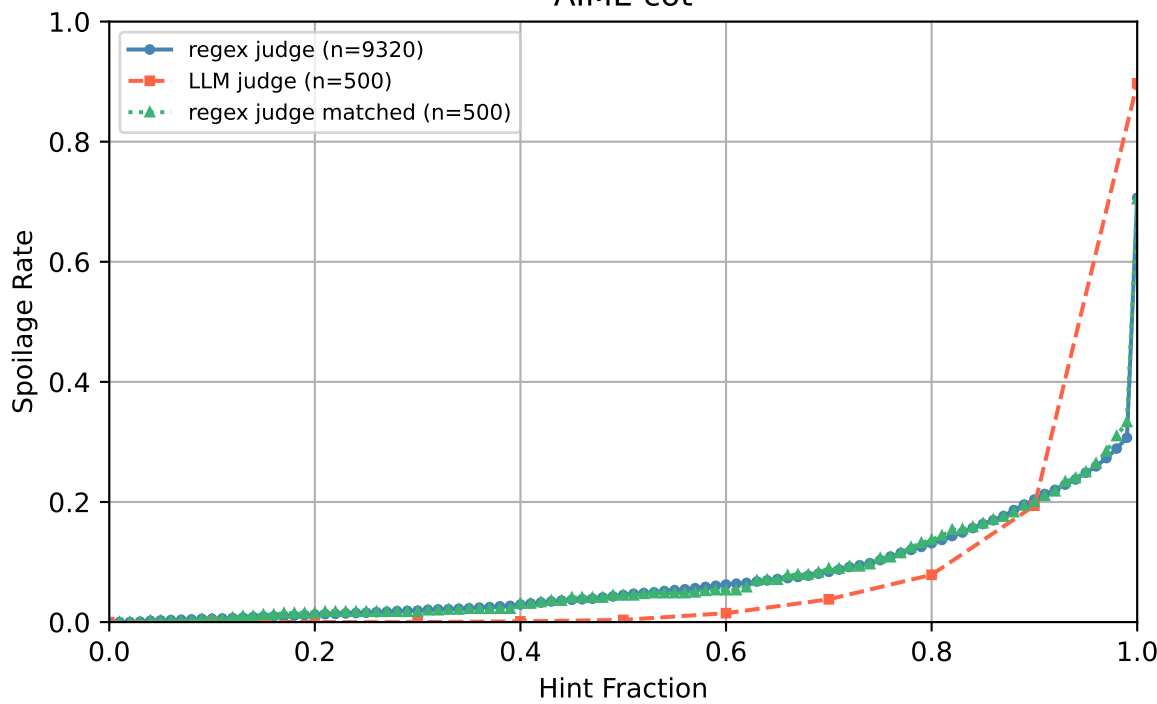
AIME cot
