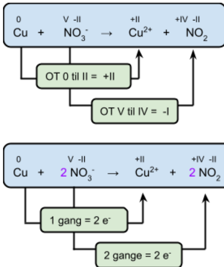
Figure 3: Trin 3: koefficienter bestemmes ud fra elektronbalancen mellem Cu og N
