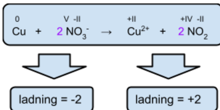
Figure 4: Trin 4: ladning = -2 på venstre side og ladning = +2 på højre side
