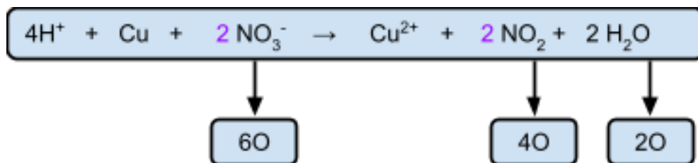
Figure 6: Trin 6: kontroltælling af 6 oxygenatomer på venstre side, 4+2 på højre side
