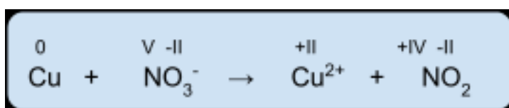
Figure 2: Trin 2: oxidationstal sat på Cu, N og O i reaktionsskemaet
