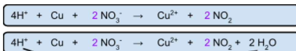
Figure 5: Trin 5: 4\text{H}^+ tilføjes på venstre side, 2\text{H}_2\text{O} dannes på højre side
