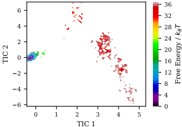
FES (TICA lag=10)
