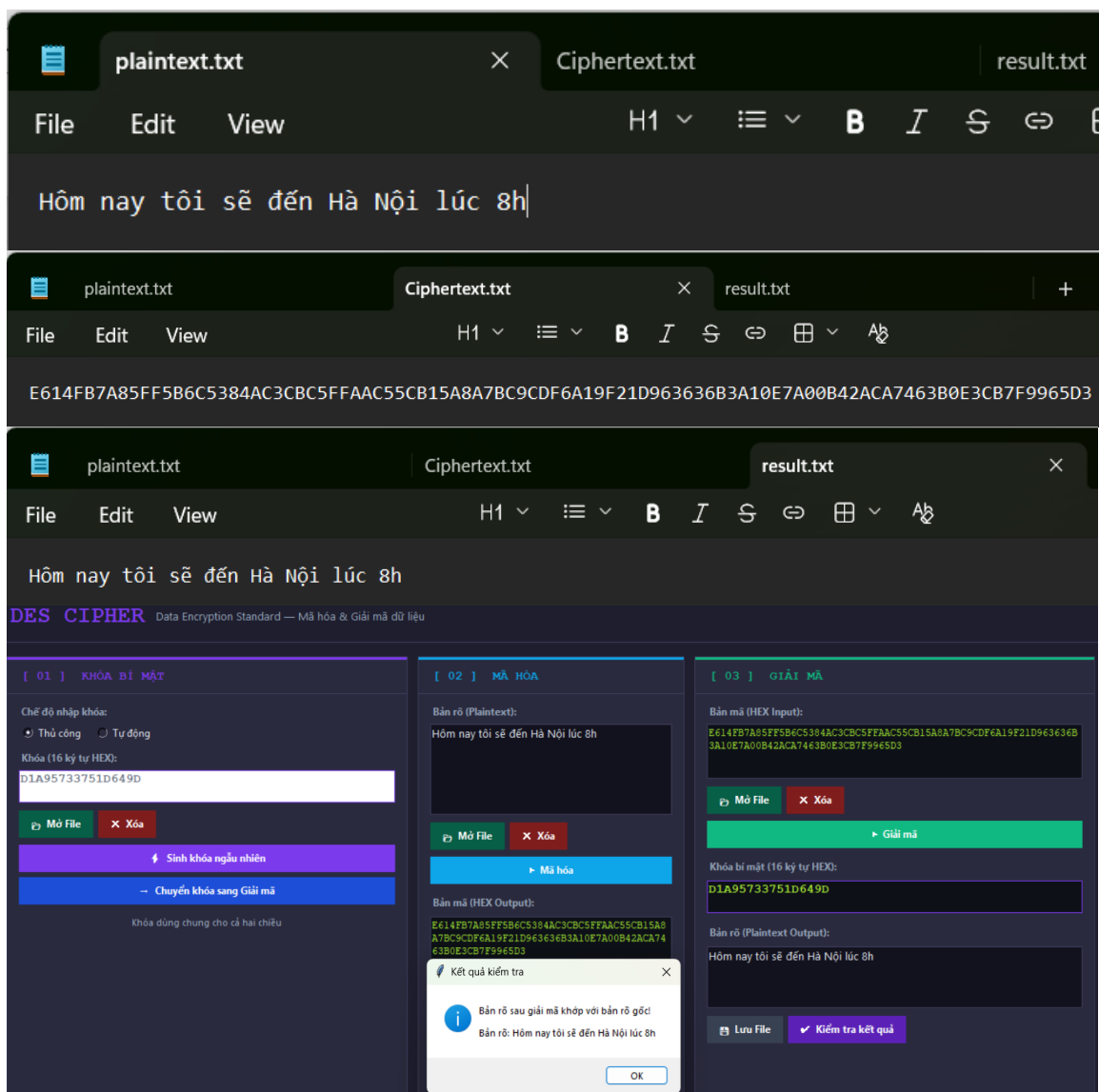
Hình 2.16: Kết quả kịch bản 4
