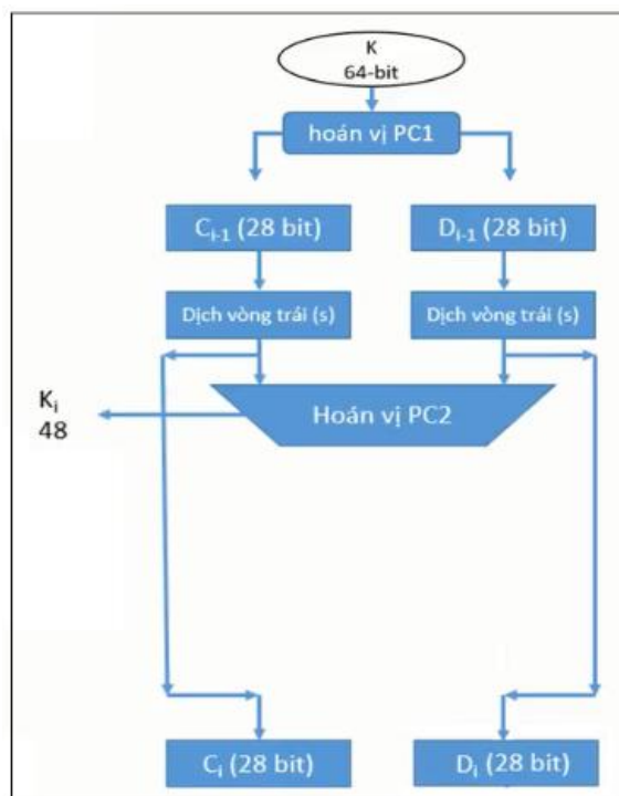
Hình 1.11: Sơ đồ quá trình sinh khóa con
