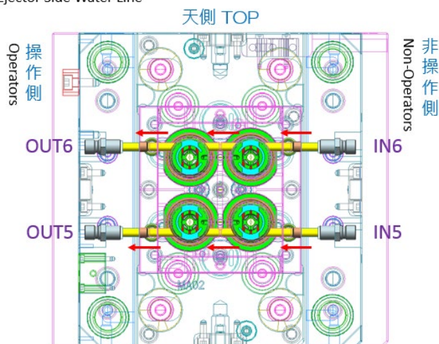
公模側水路分佈圖
