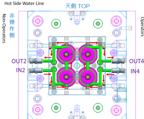
母模側水路分佈圖 1
