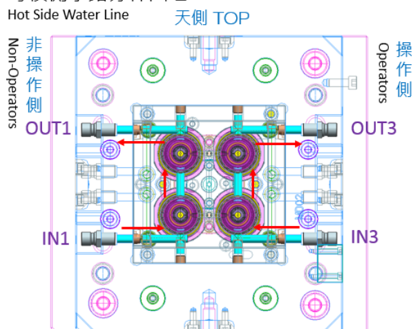
母模側水路分佈圖 2
