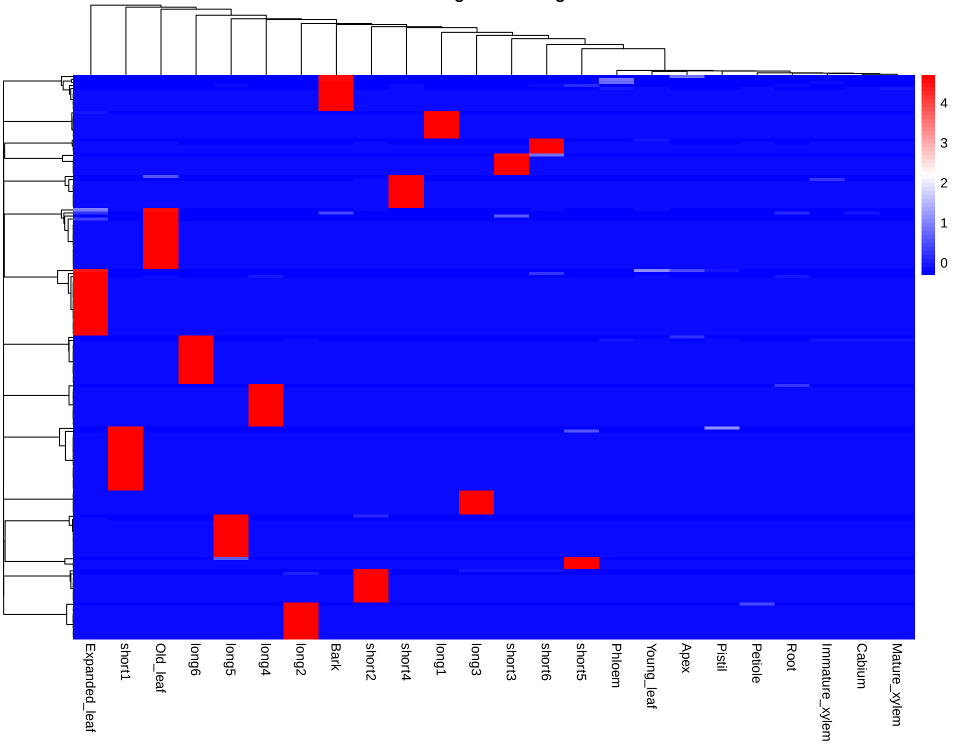
Module: green – 186 genes
