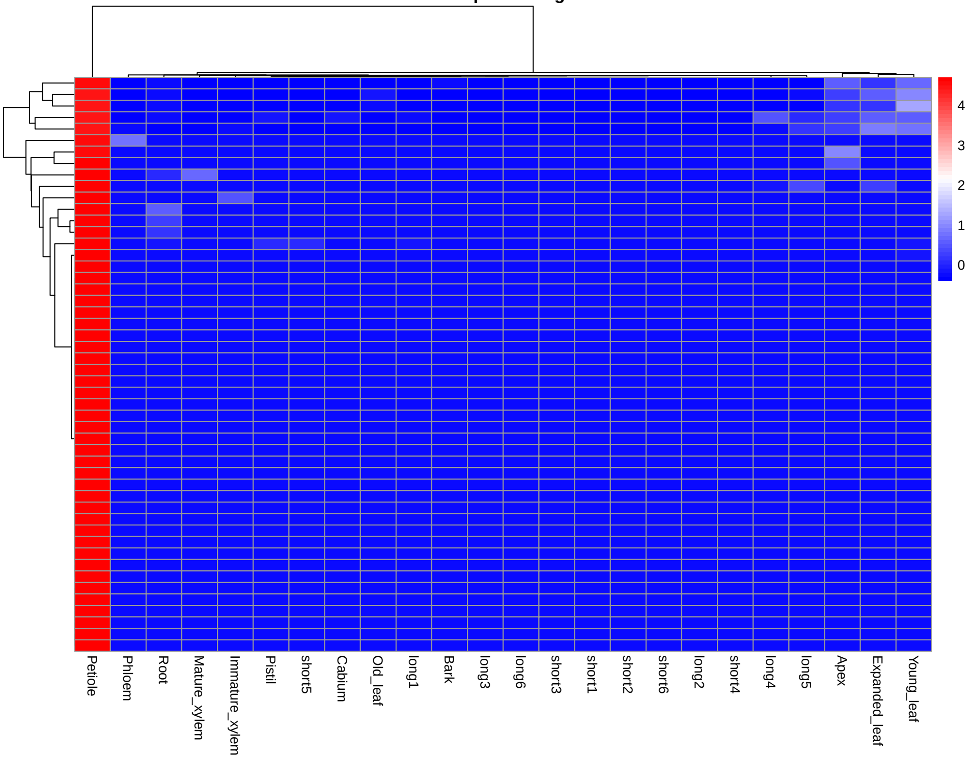
Module: pink - 50 genes
