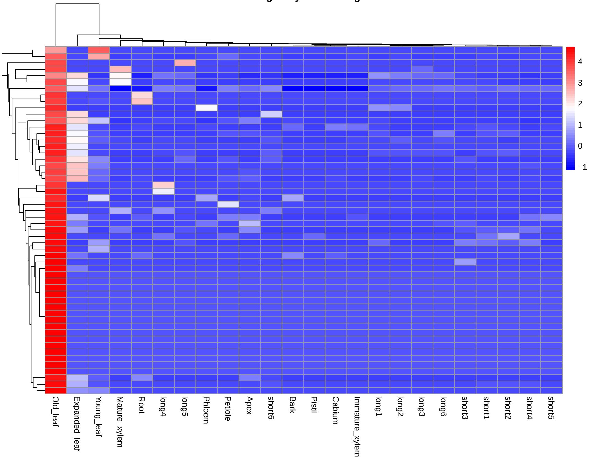
Module: greenyellow - 54 genes
