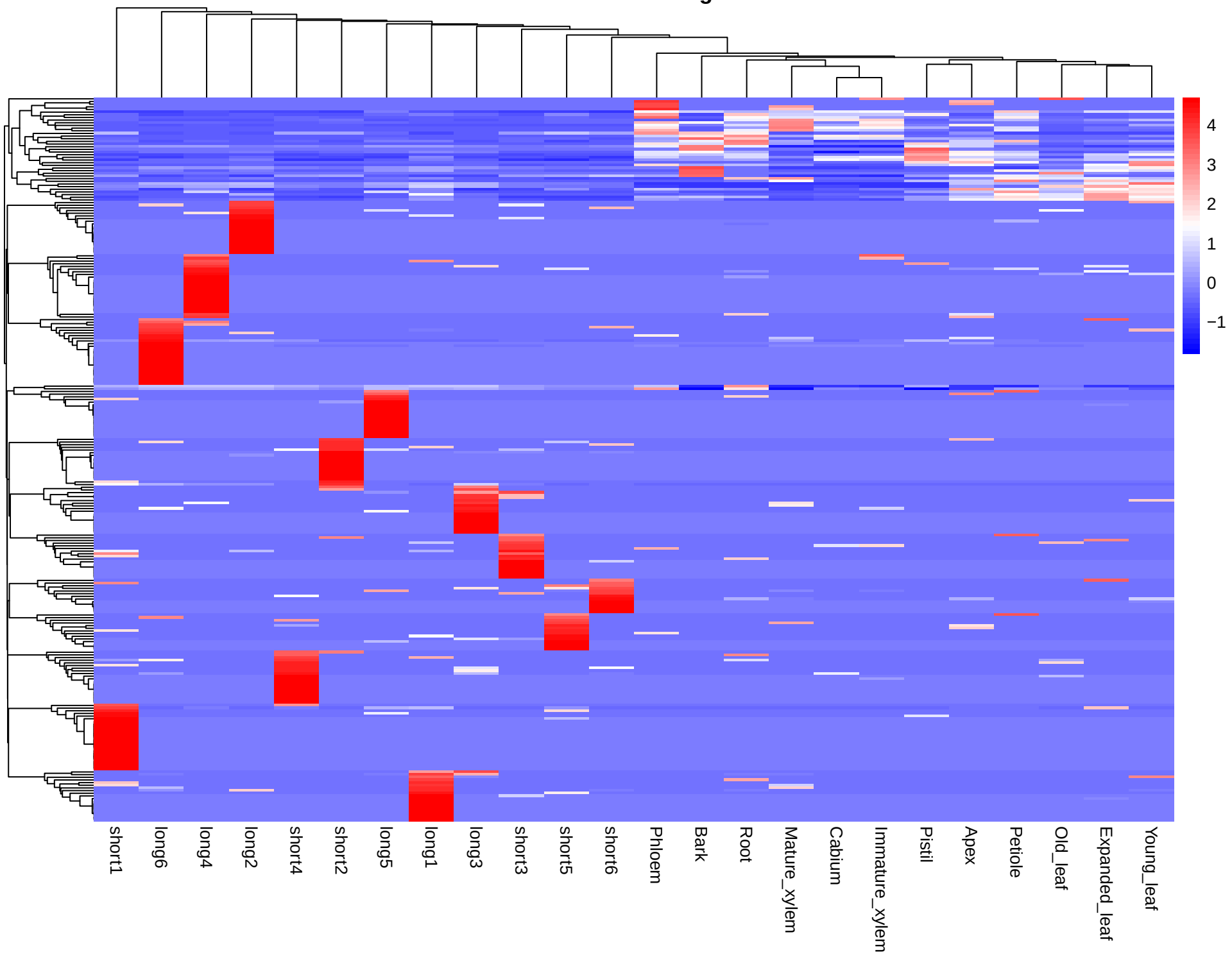
Module: red - 272 genes
