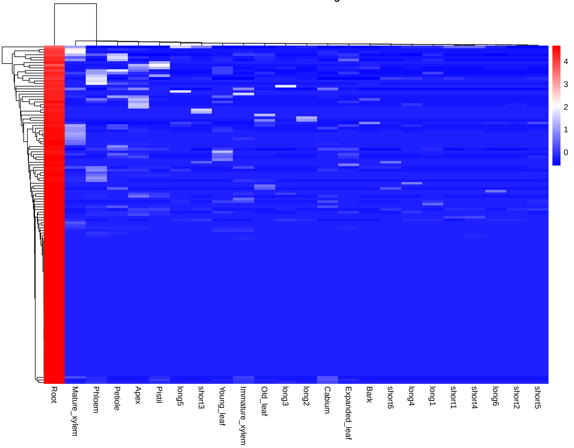
Module: brown - 129 genes
