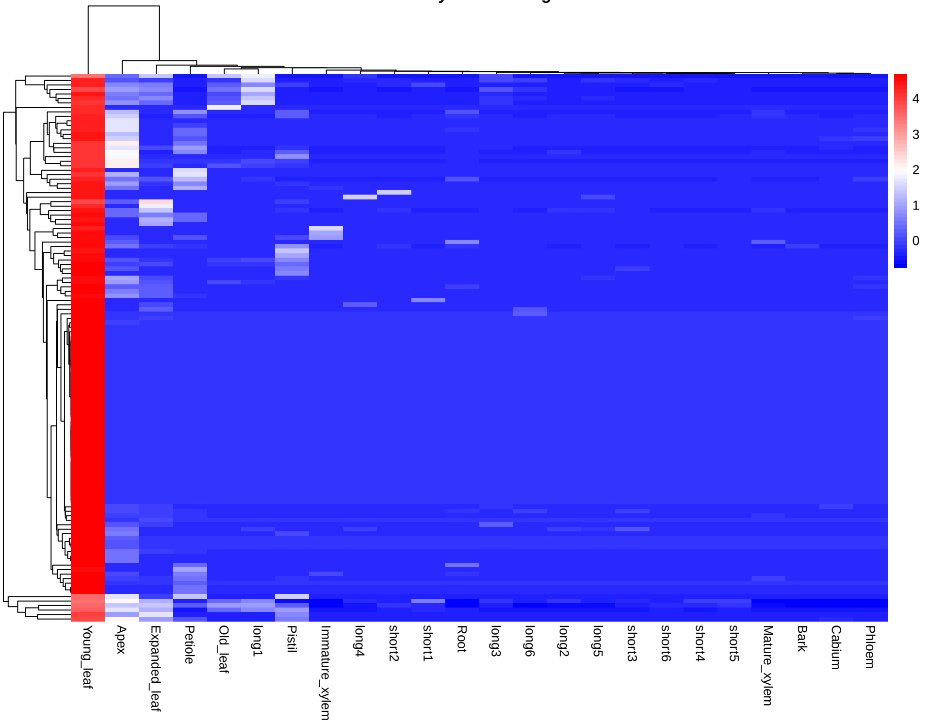
Module: yellow – 122 genes
