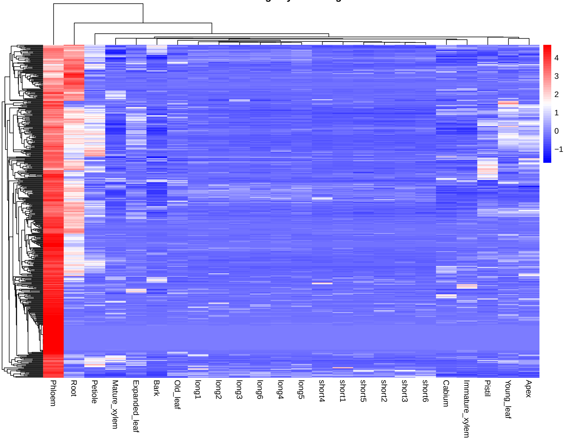
Module: lightcyan – 480 genes
