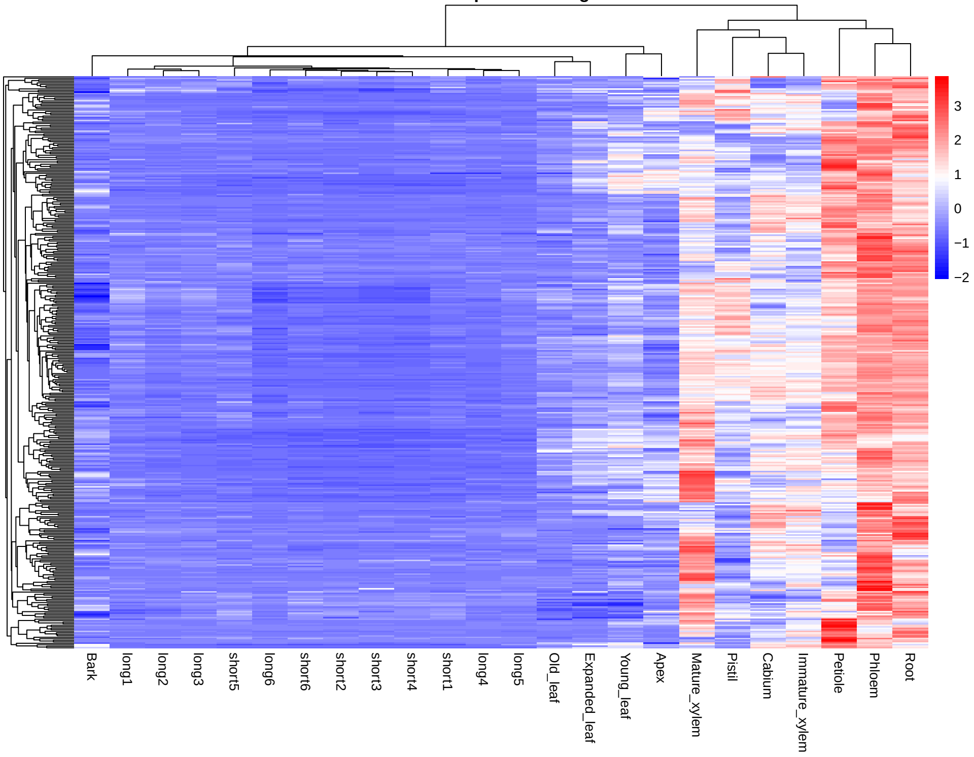
Module: turquoise - 380 genes
