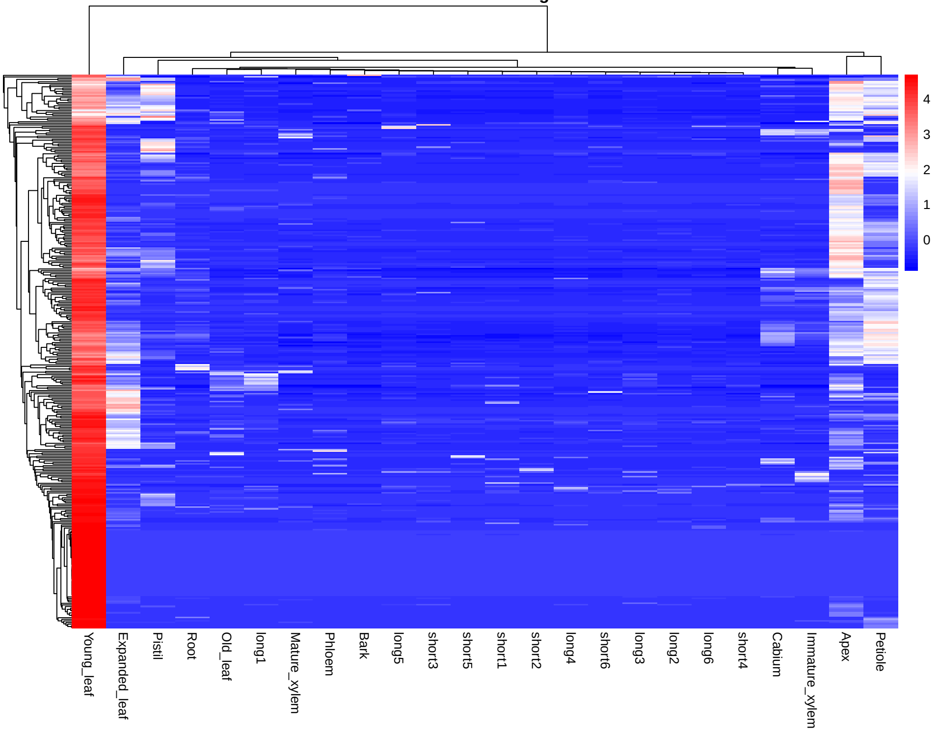
Module: blue - 346 genes
