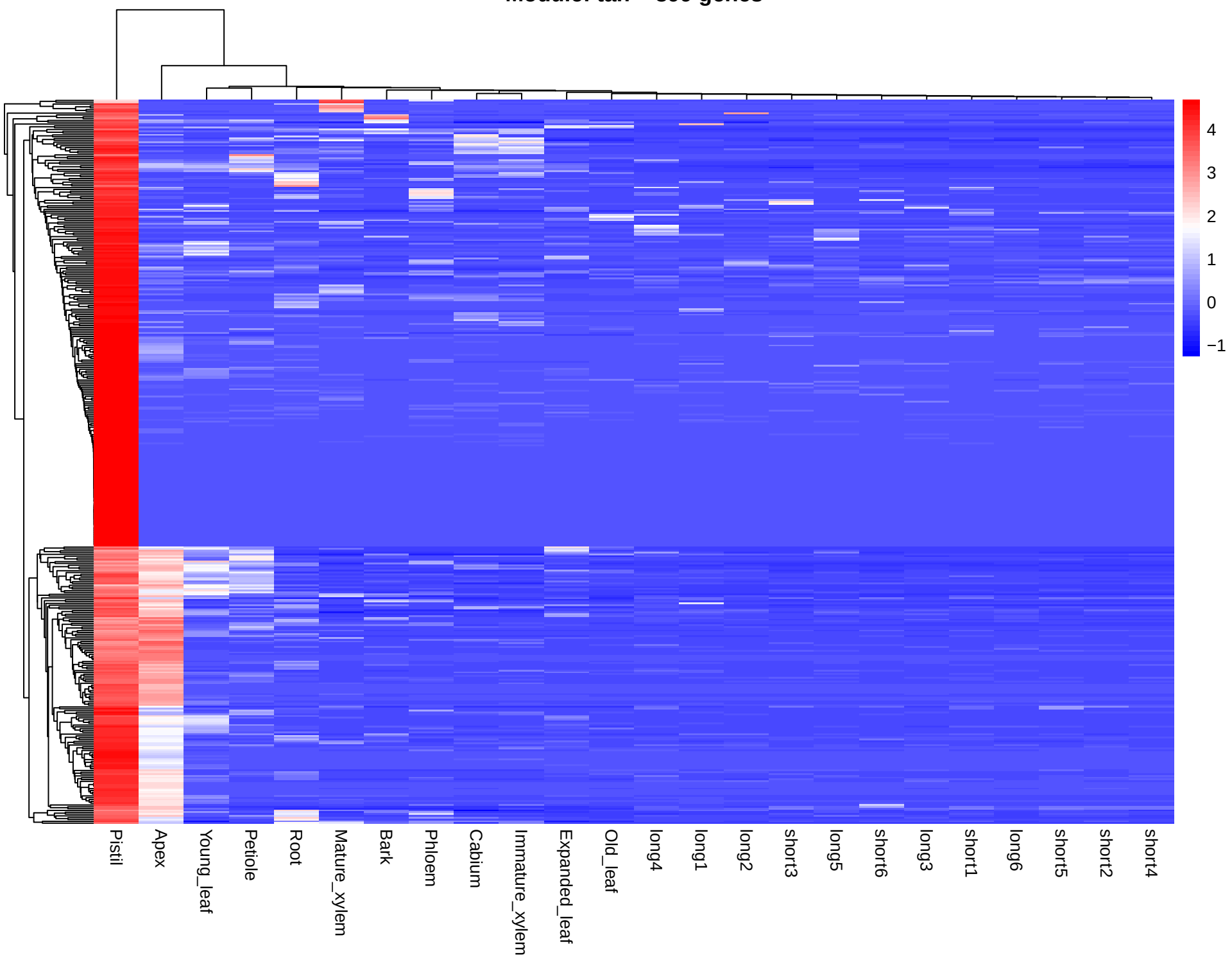
Module: tan - 399 genes
