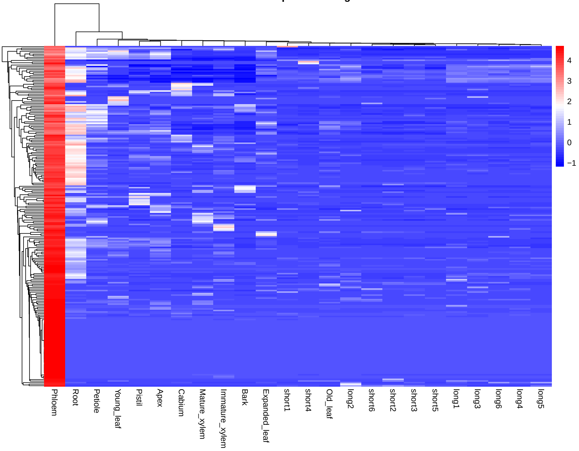
Module: turquoise - 222 genes
