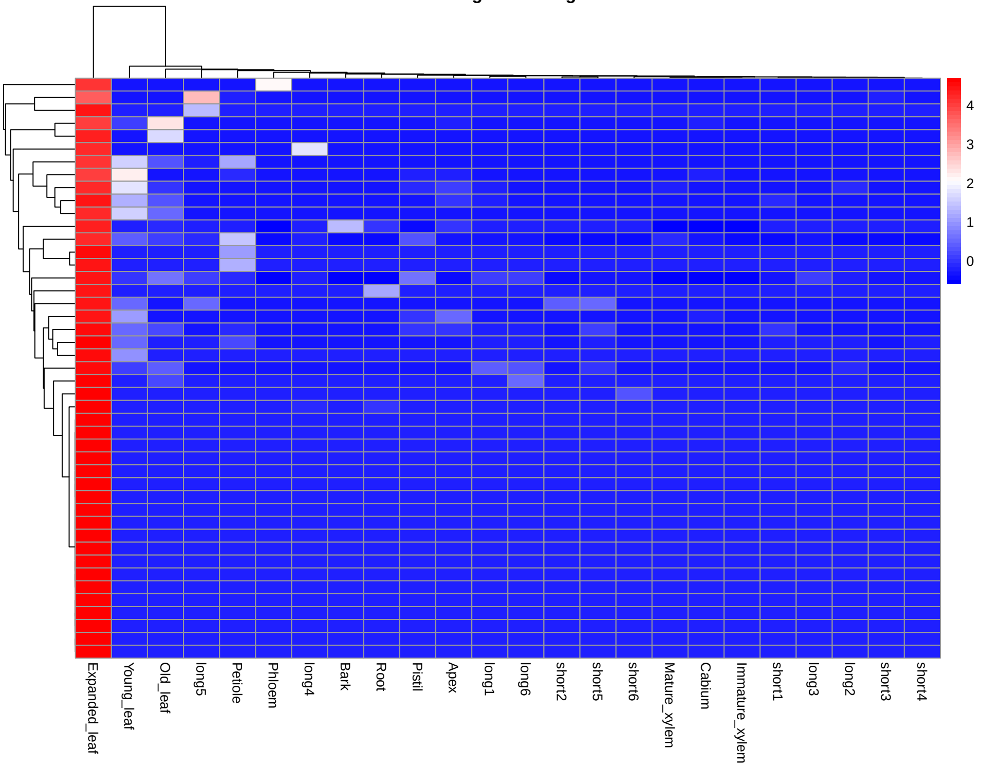
Module: green - 45 genes
