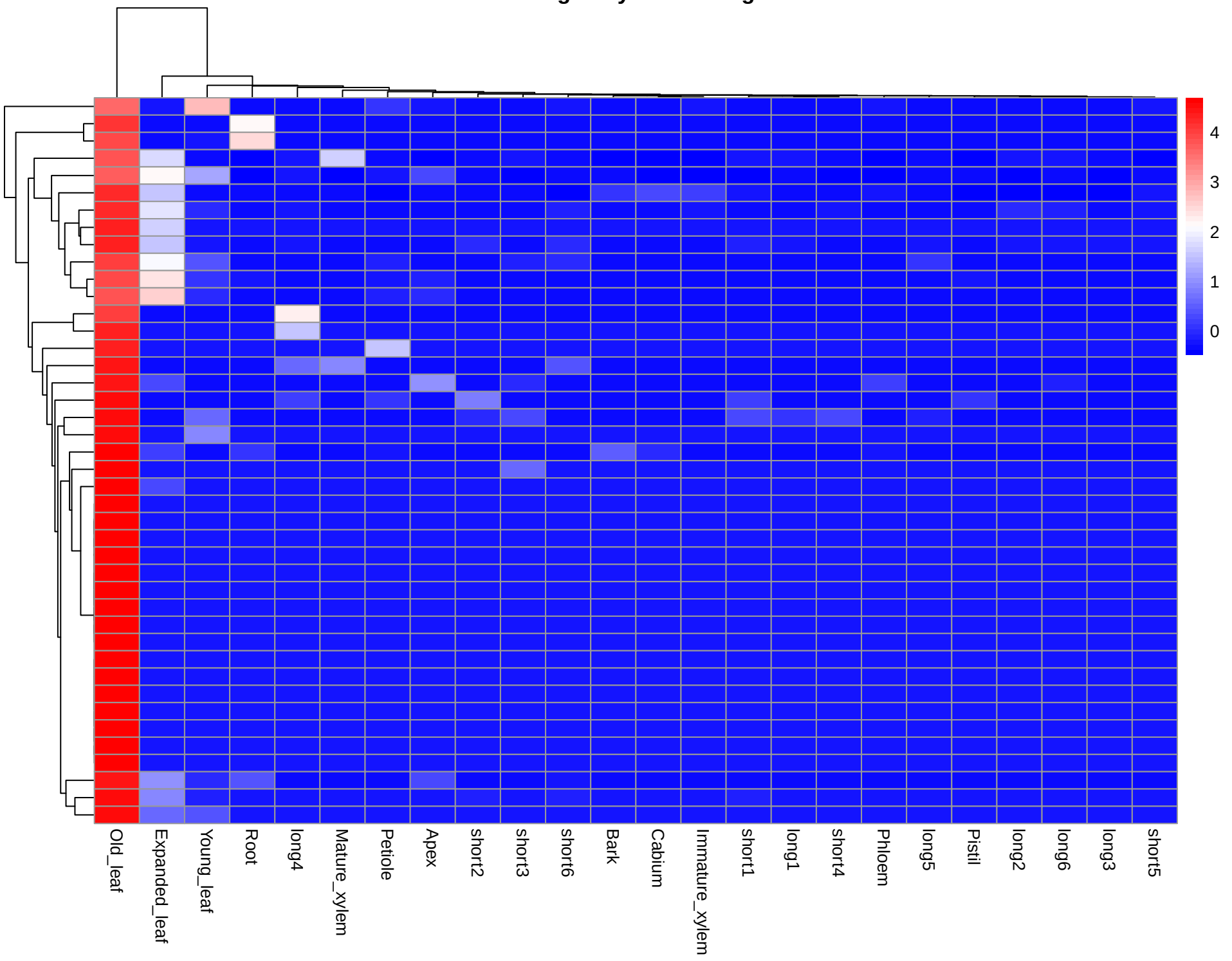
Module: greenyellow – 42 genes
