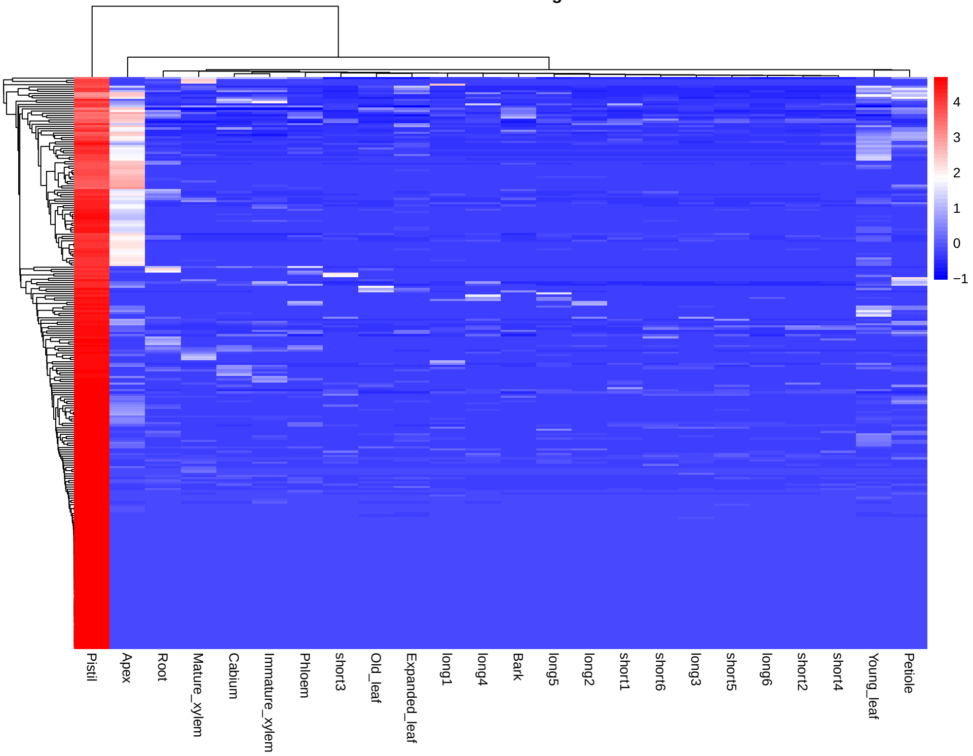
Module: tan - 260 genes
