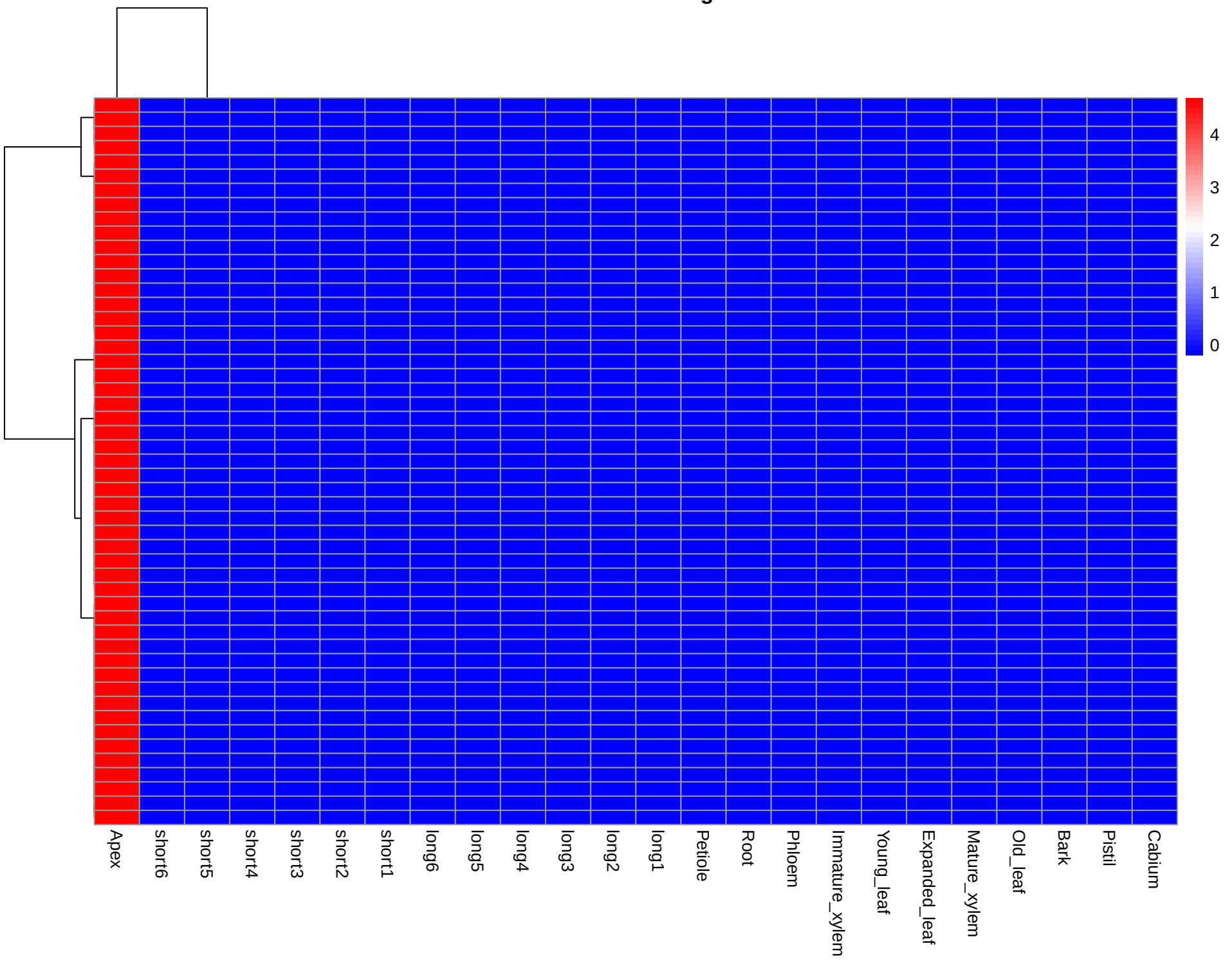
Module: blue – 51 genes
