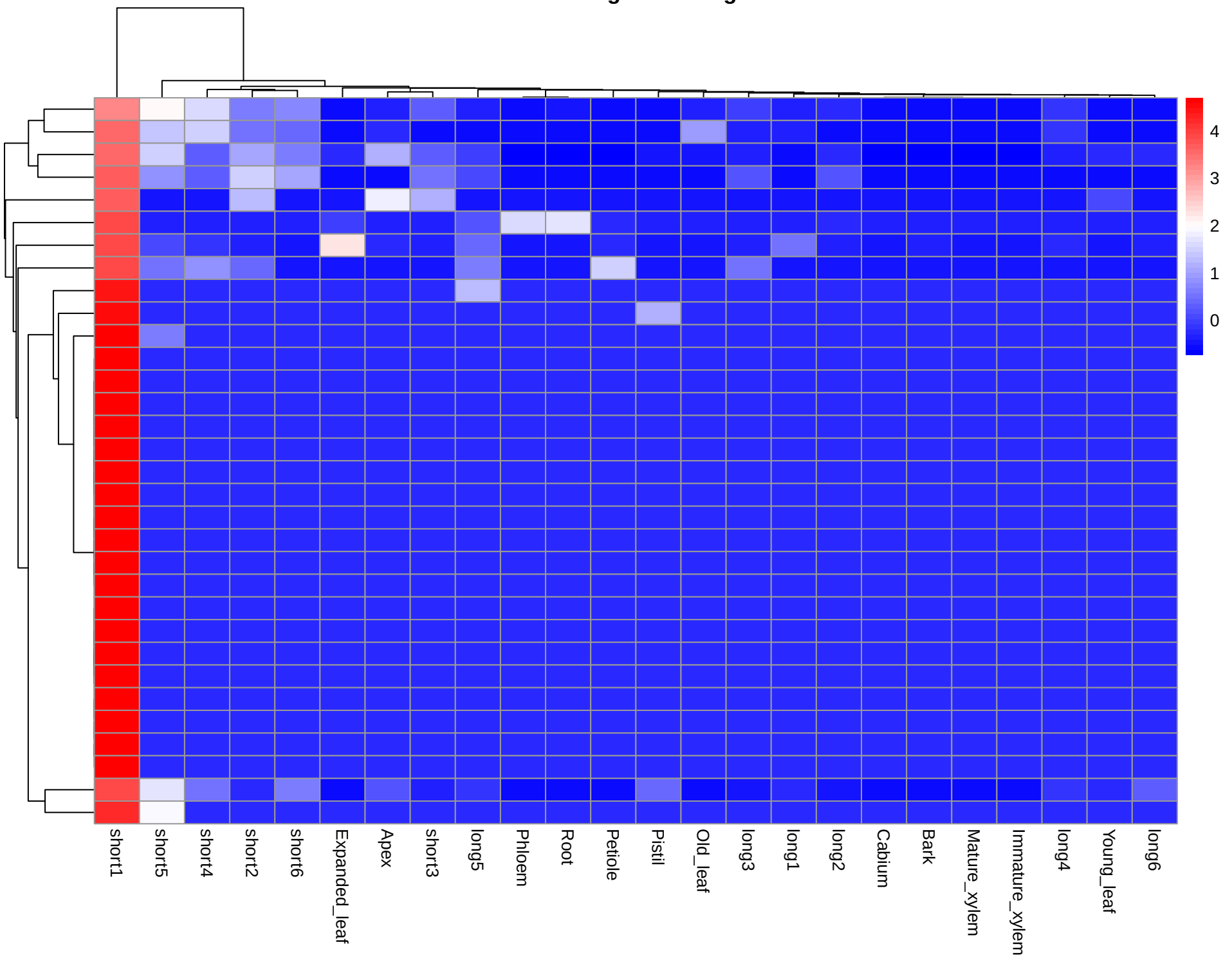
Module: magenta – 32 genes
