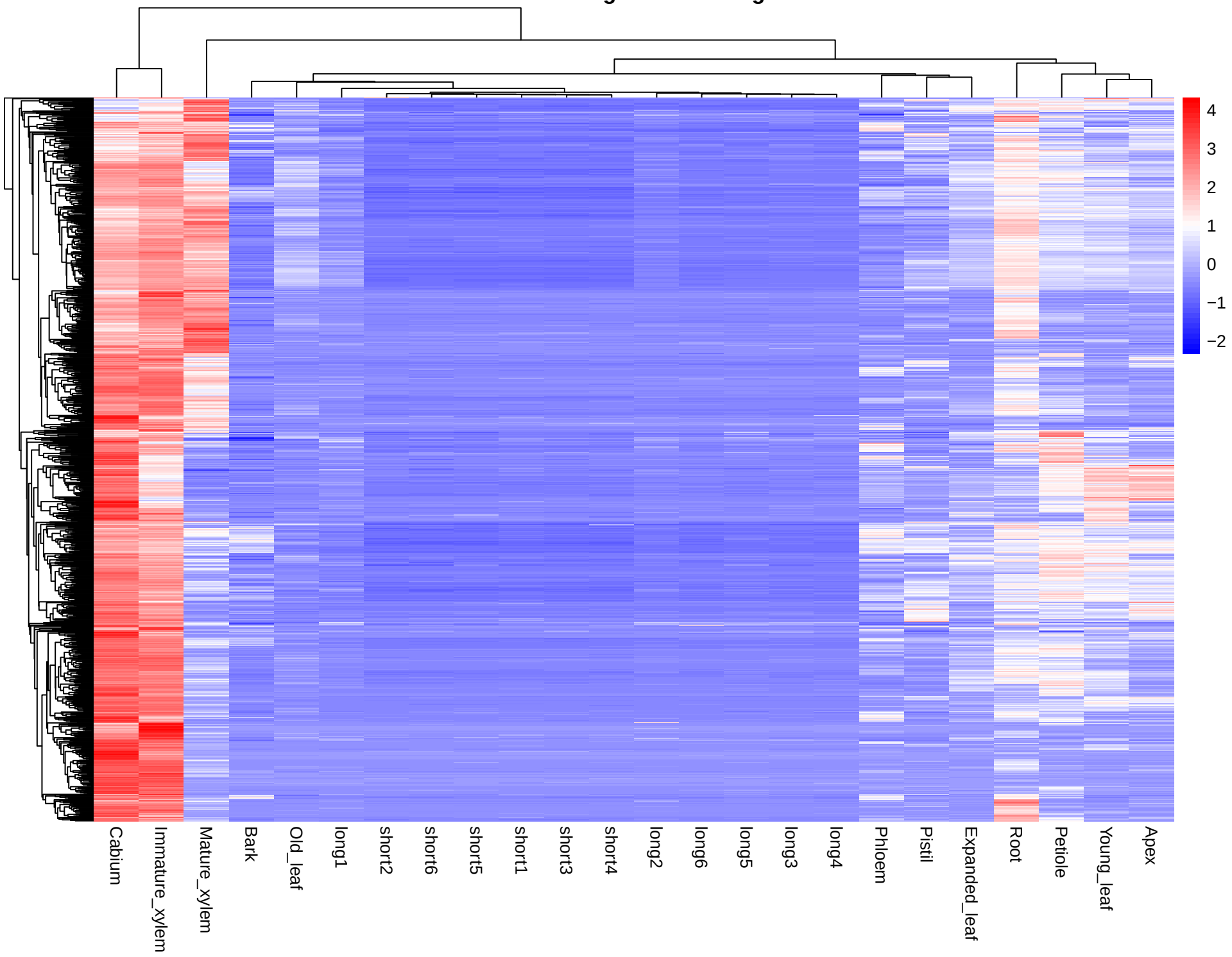
Module: midnightblue - 932 genes
