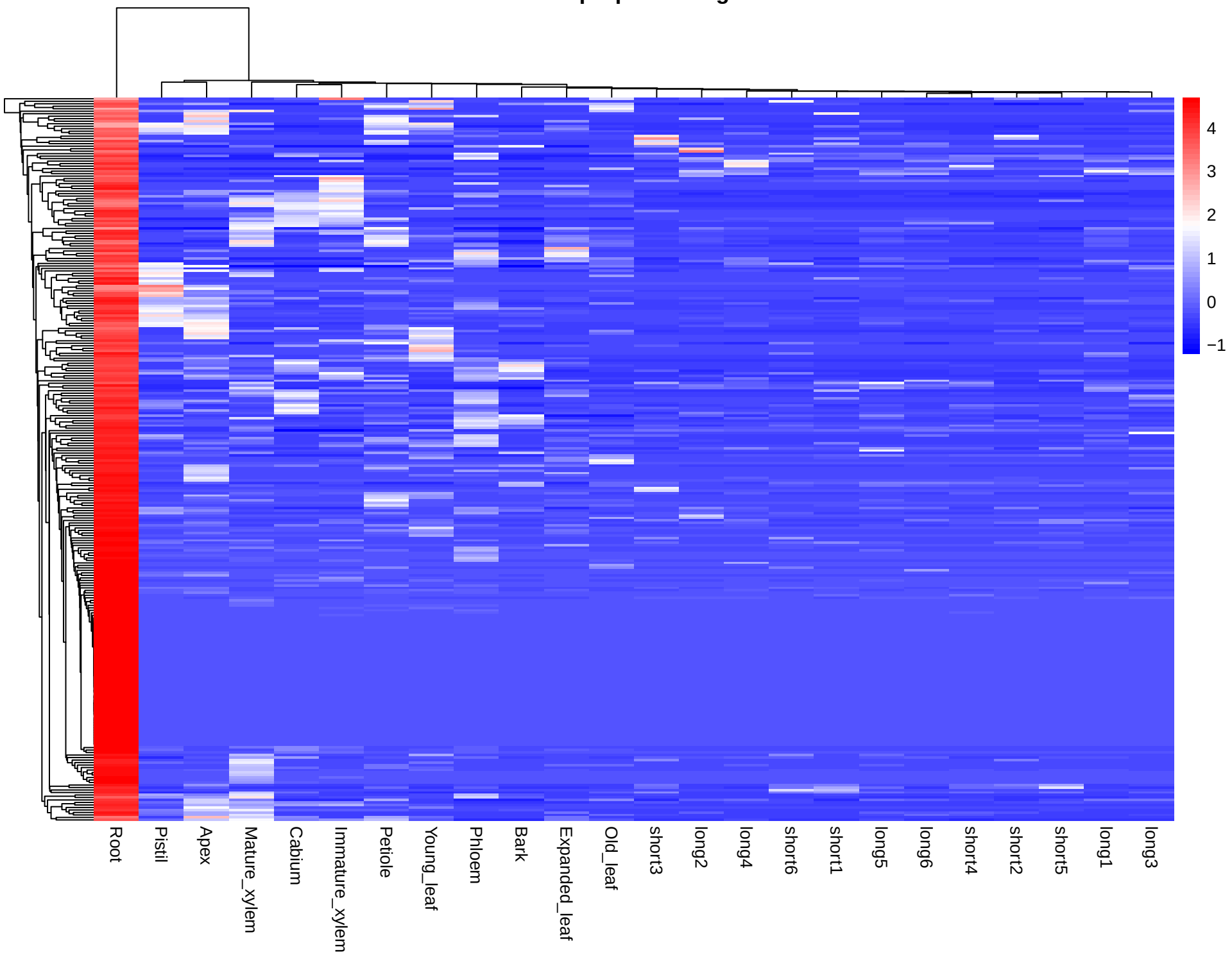
Module: purple – 290 genes
