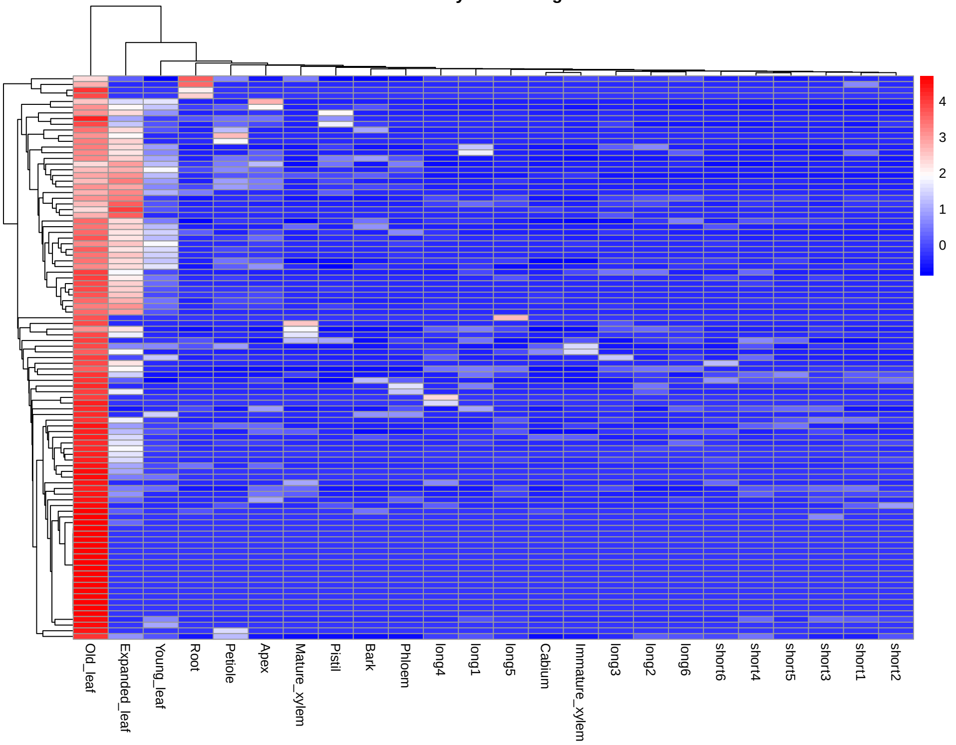
Module: yellow – 99 genes
