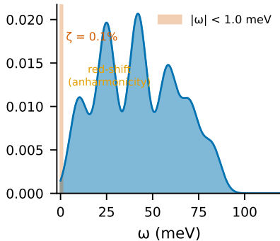
(b) Anharmonic VDOS (VACF)
