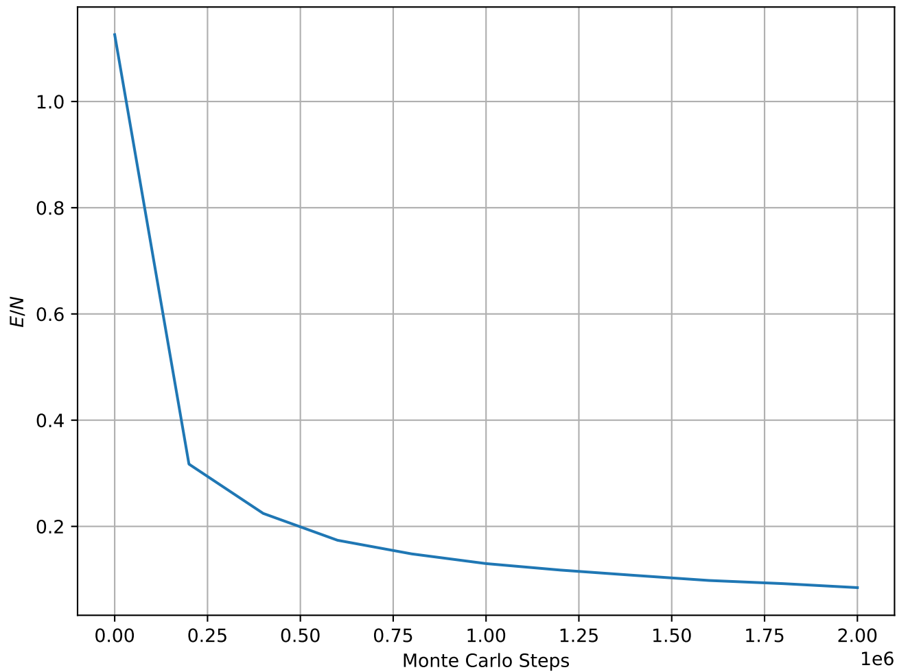
Energy per Spin at T = 1.00e - 02 , L = 64
