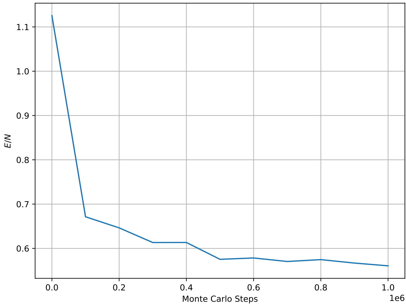
Energy per Spin at T = 1.75e - 01 , L = 64
