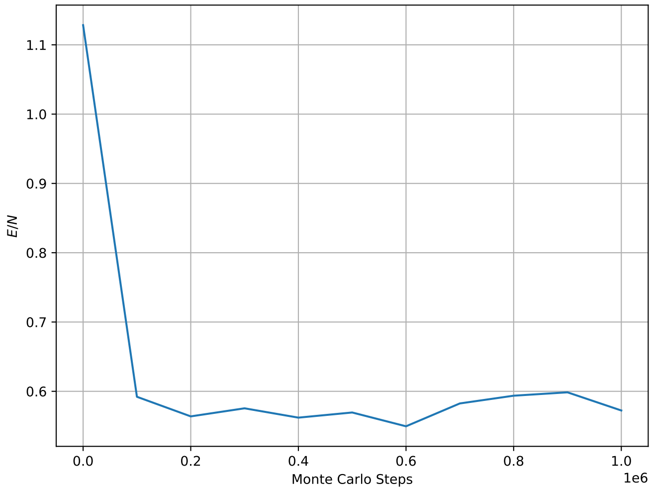
Energy per Spin at T = 1.80e - 01 , L = 32
