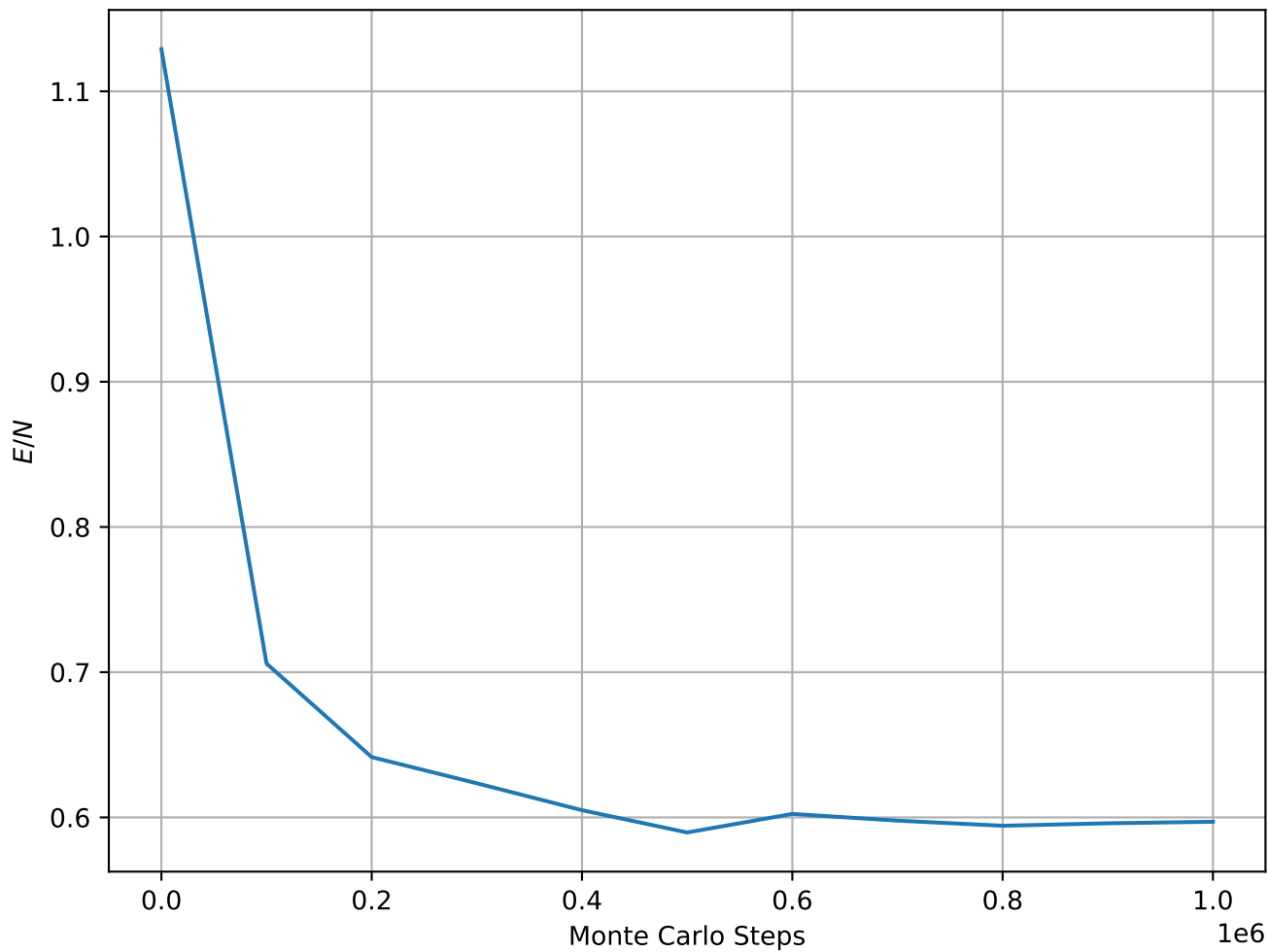
Energy per Spin at T = 1.8e - 01 , L = 64
