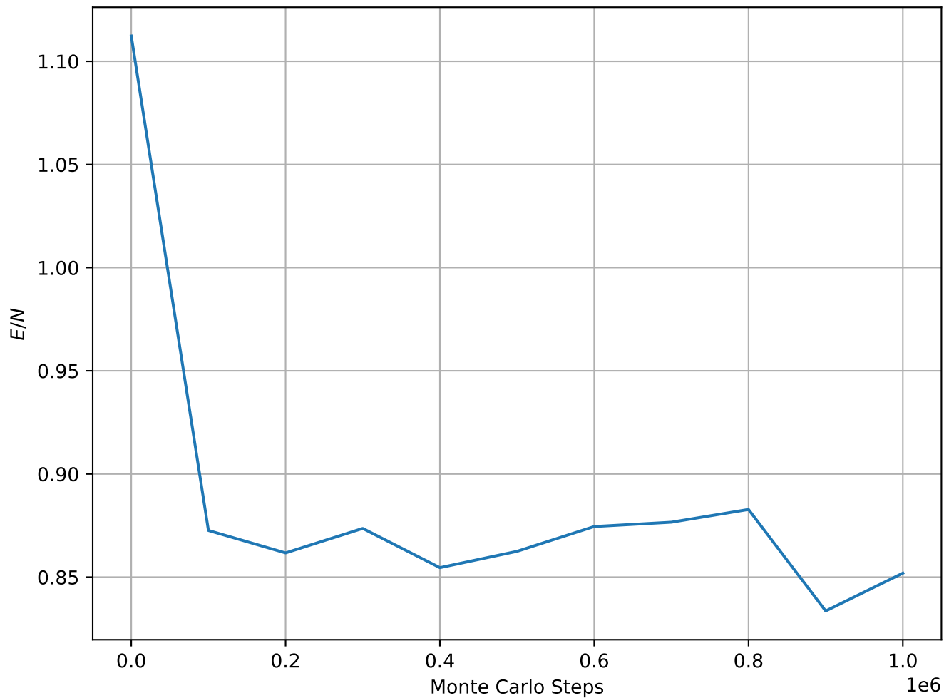
Energy per Spin at T = 2.50e - 01 , L = 32
