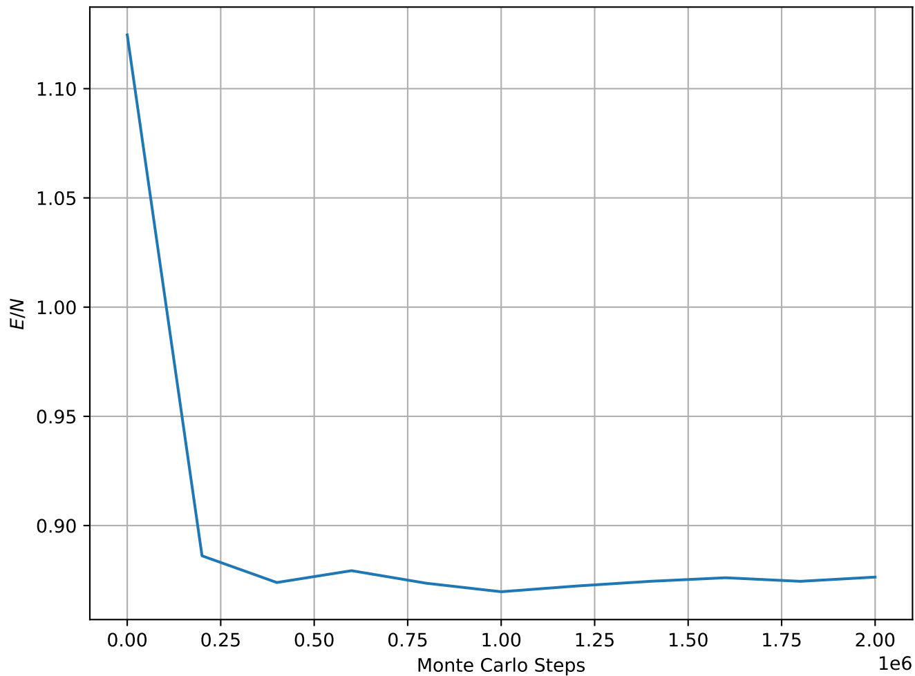
Energy per Spin at T = 2.50e - 01 , L = 64
