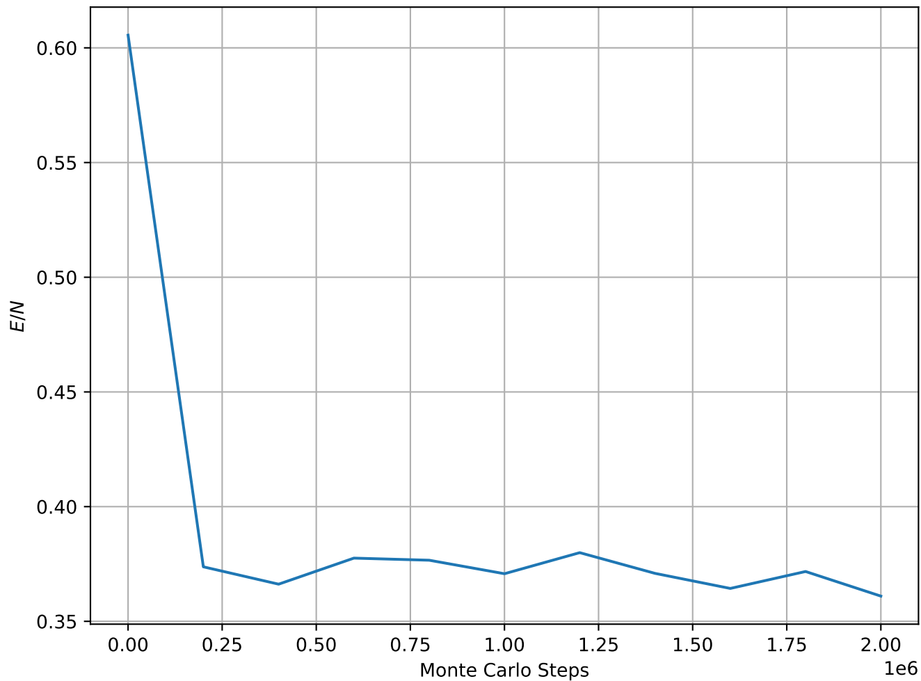
Energy per Spin at T = 1.20e - 01 , L = 64
