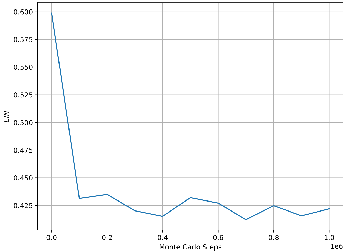
Energy per Spin at T = 1.50e - 01 , L = 32
