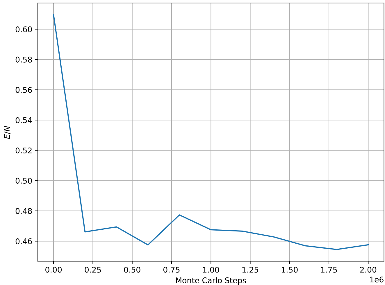
Energy per Spin at T = 1.50e - 01 , L = 64
