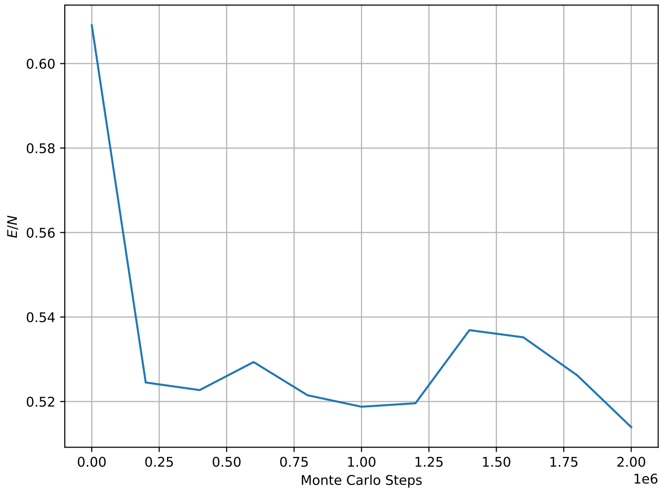
Energy per Spin at T = 1.90e - 01 , L = 64
