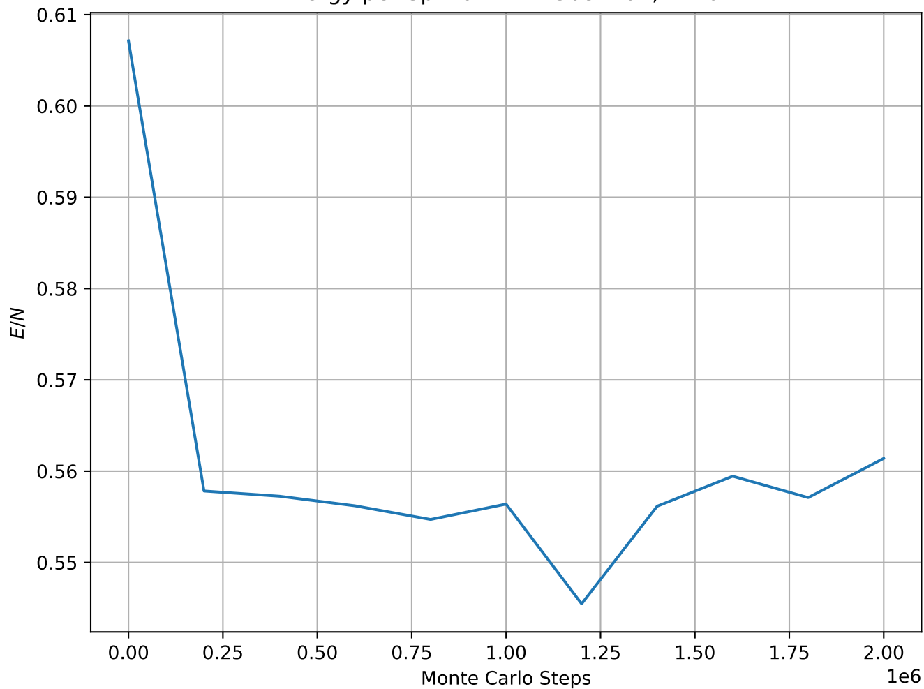
Energy per Spin at T = 2.50e - 01 , L = 64
