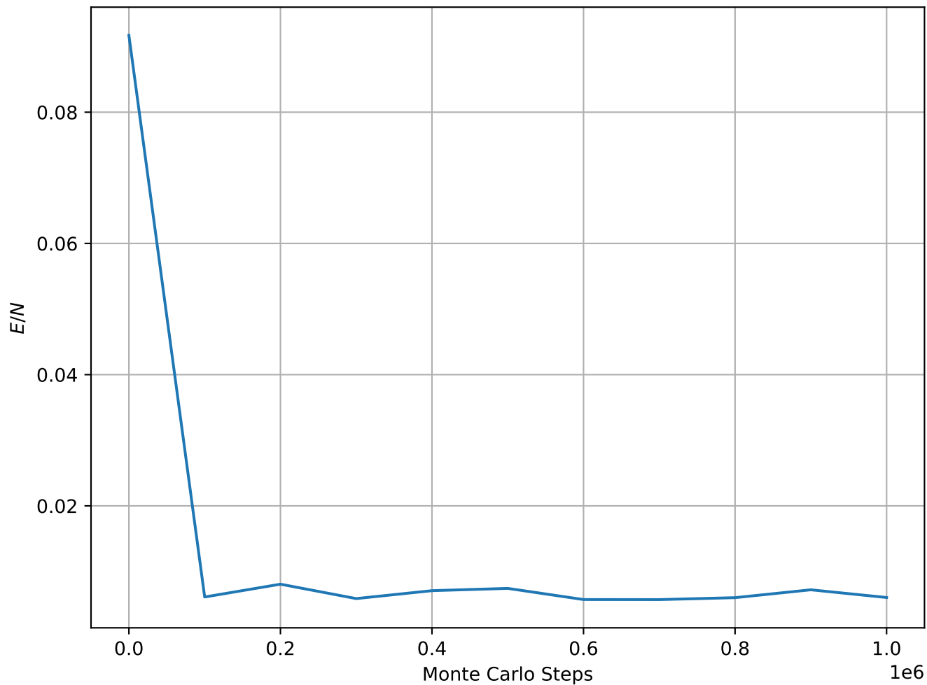
Energy per Spin at T = 1.0e - 02 , L = 64
