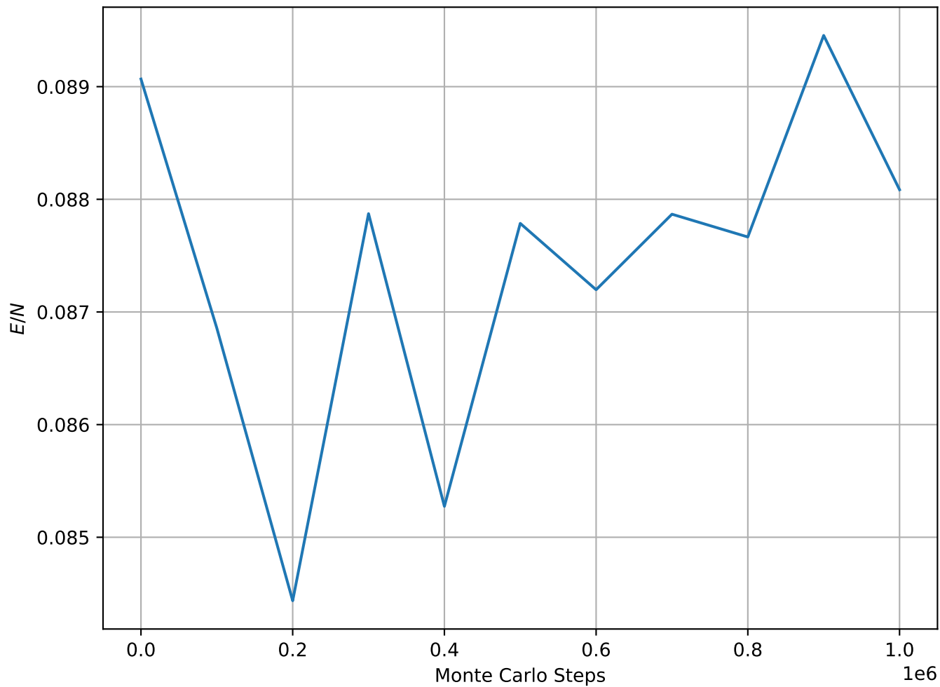
Energy per Spin at T = 1.5e - 01 , L = 64
