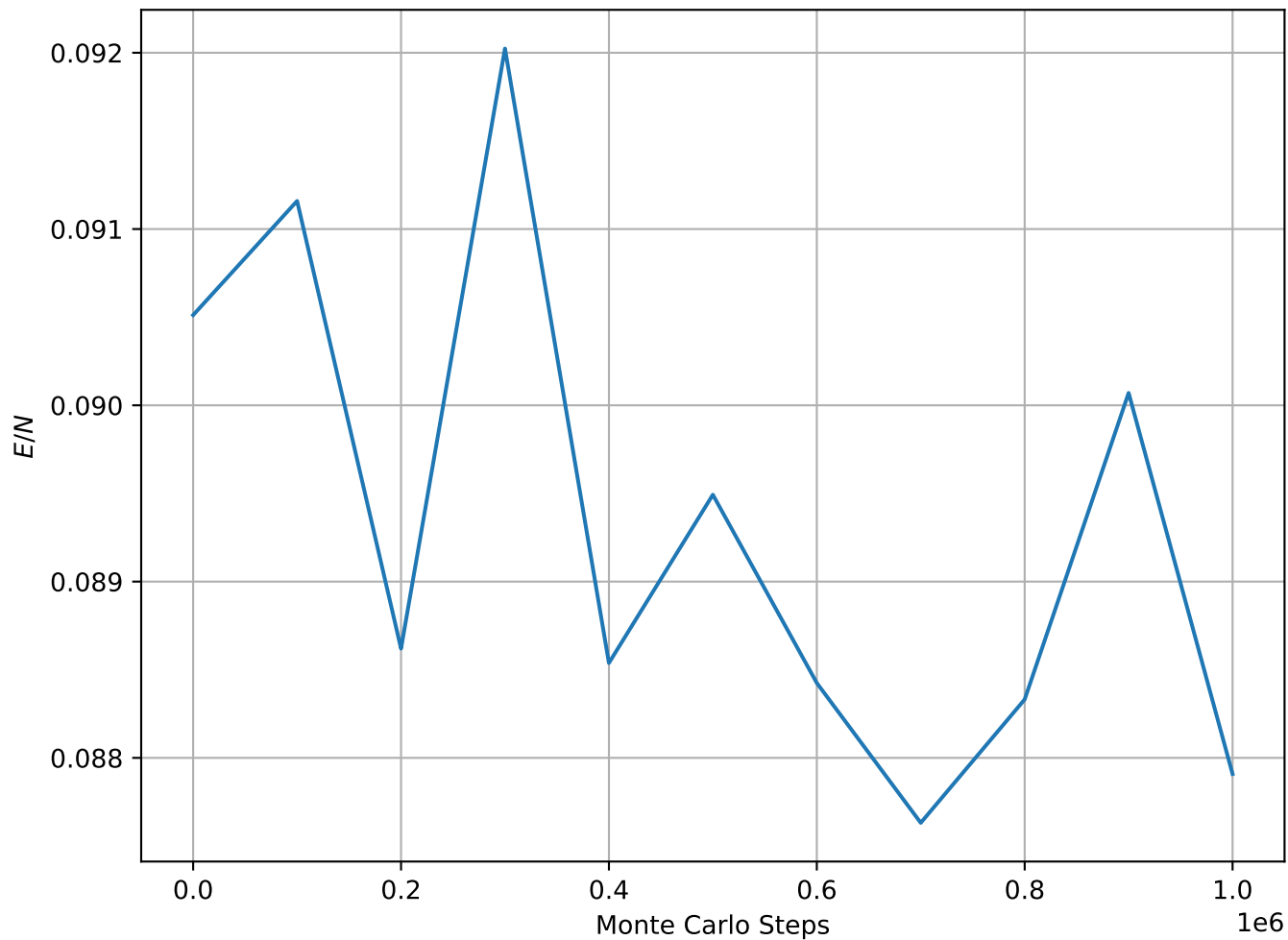
Energy per Spin at T = 2.0e - 01 , L = 64
