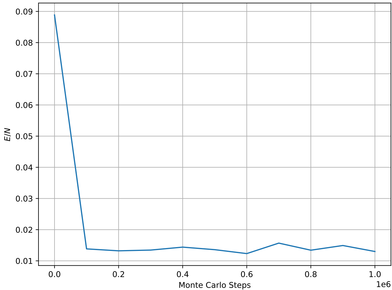
Energy per Spin at T = 2.0e - 02 , L = 64
