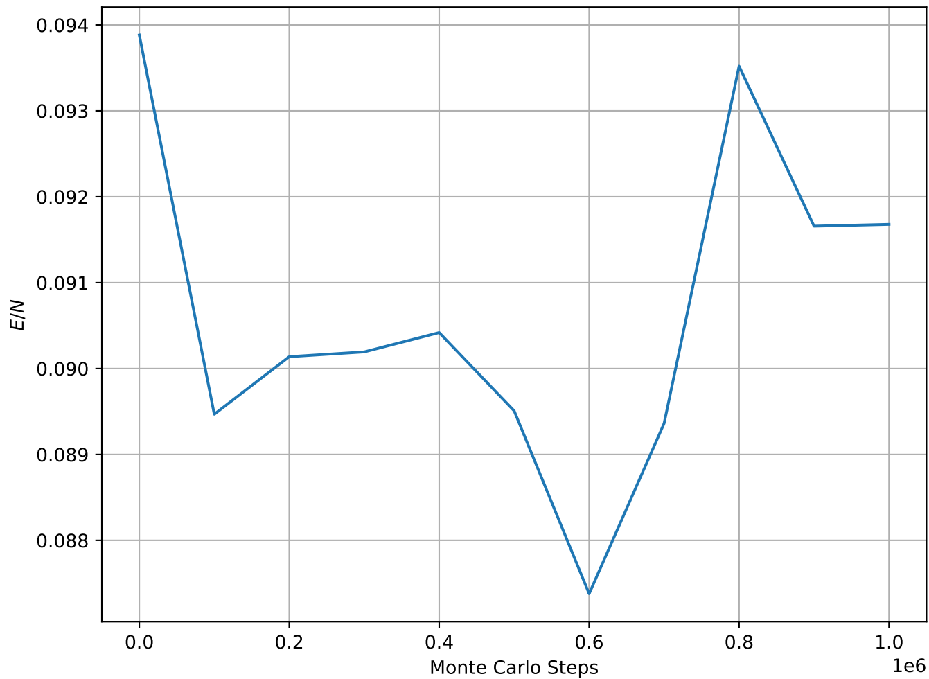
Energy per Spin at T = 2.5e - 01 , L = 64
