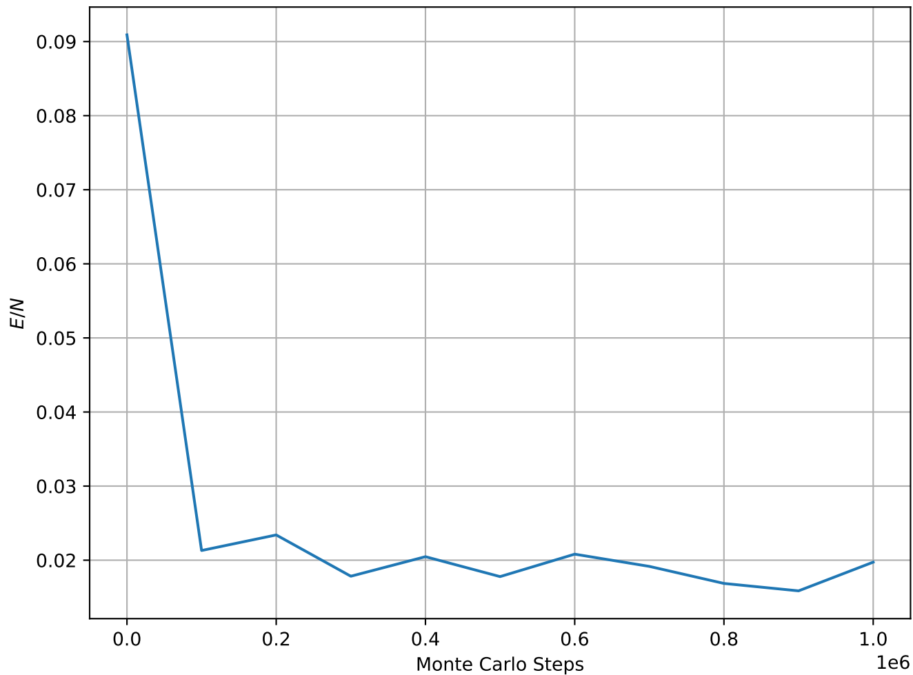
Energy per Spin at T = 3.00e - 02 , L = 32
