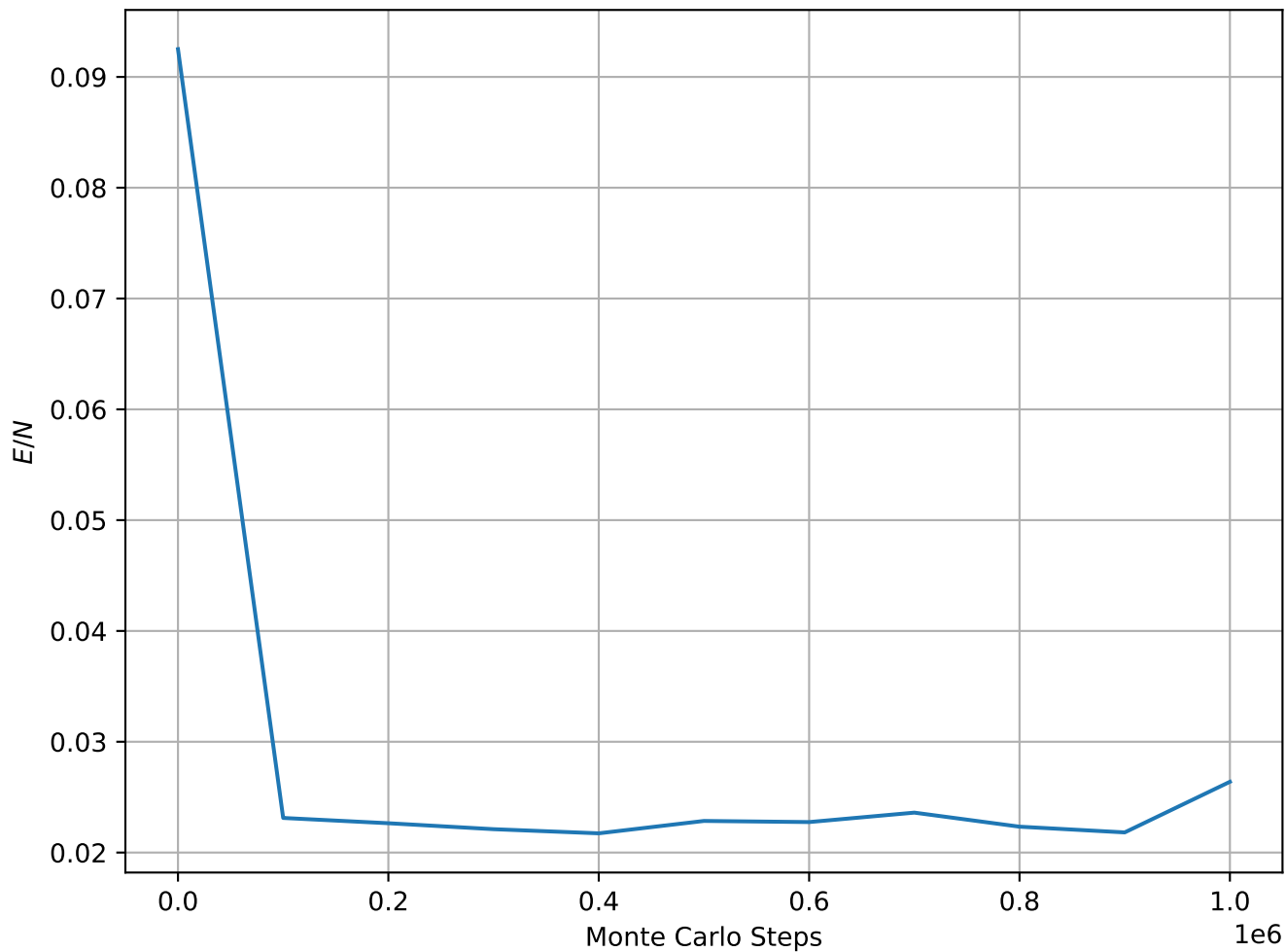
Energy per Spin at T = 3.0e - 02 , L = 64
