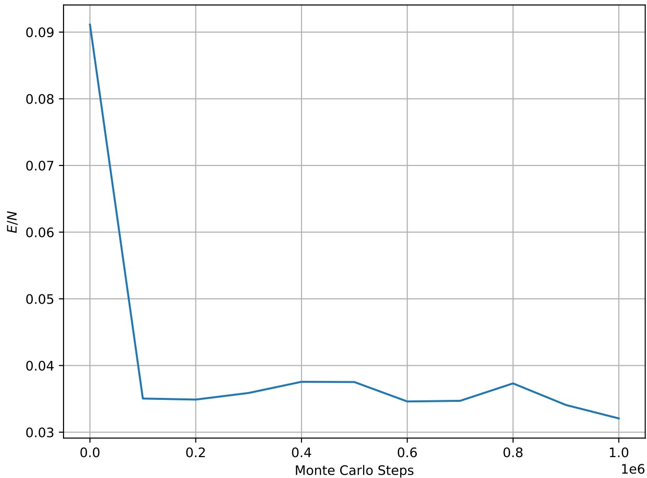
Energy per Spin at T = 4.0e - 02 , L = 64
