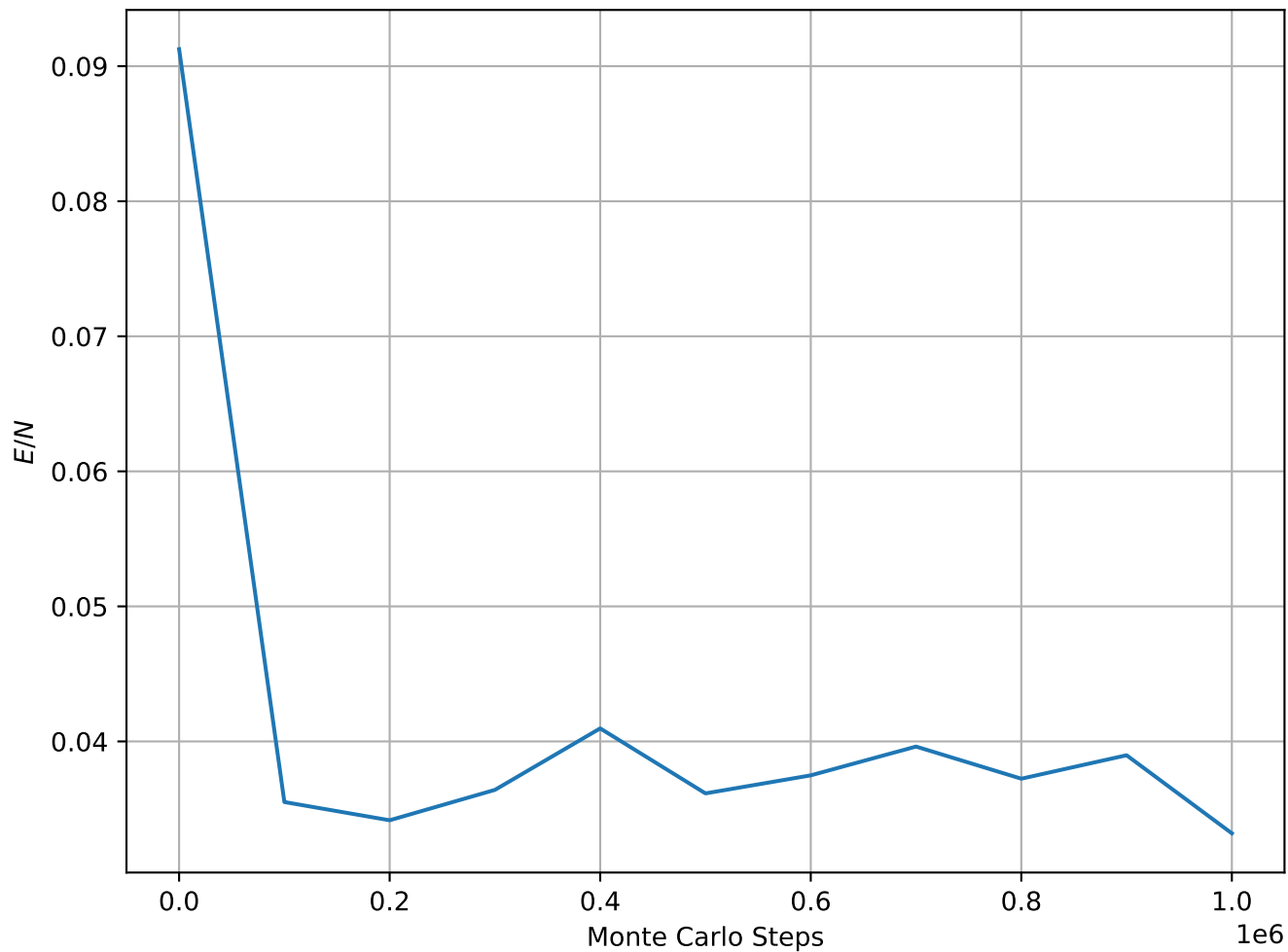
Energy per Spin at T = 5.00e - 02 , L = 32
