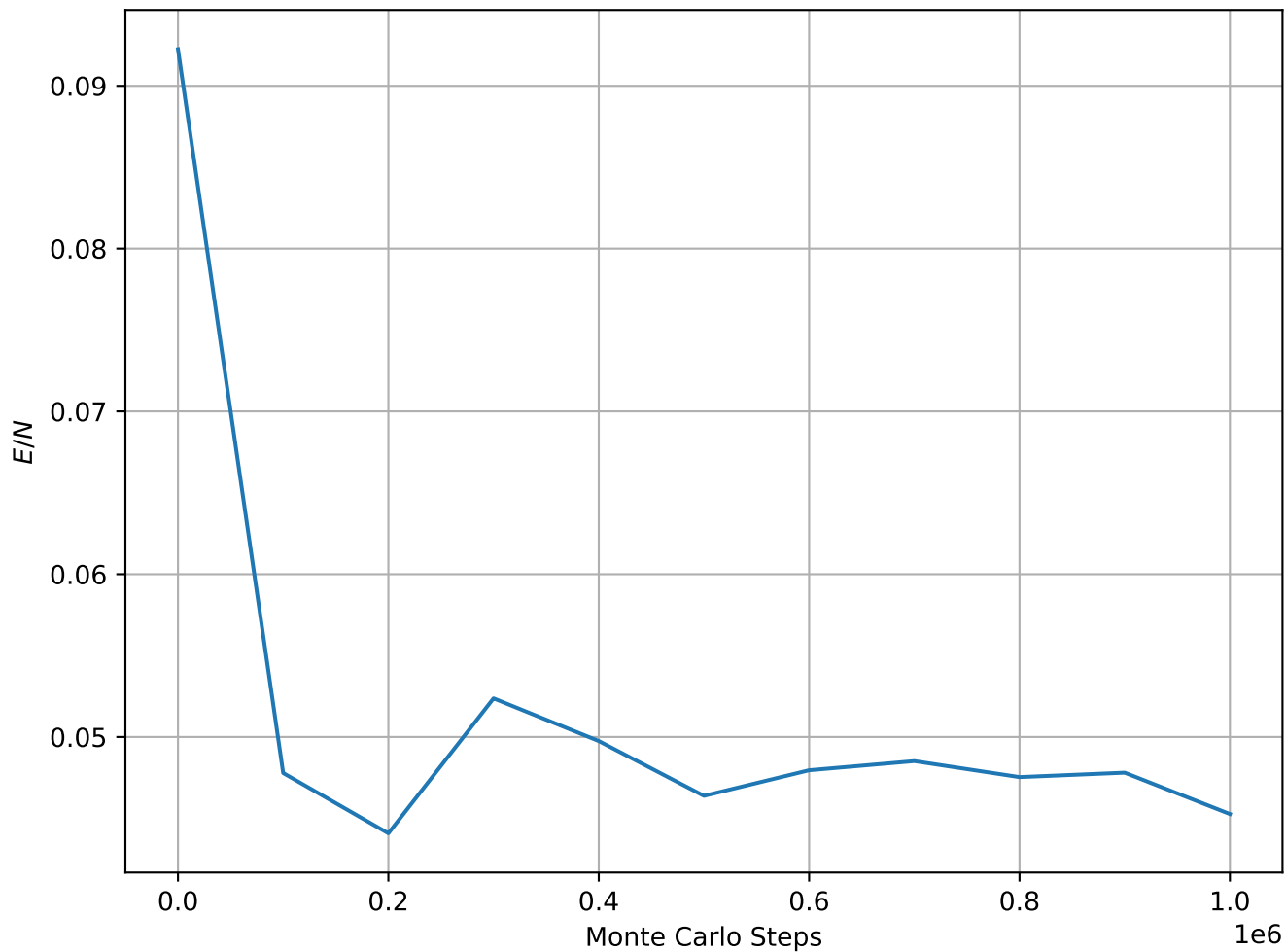
Energy per Spin at T = 5.0e - 02 , L = 64
