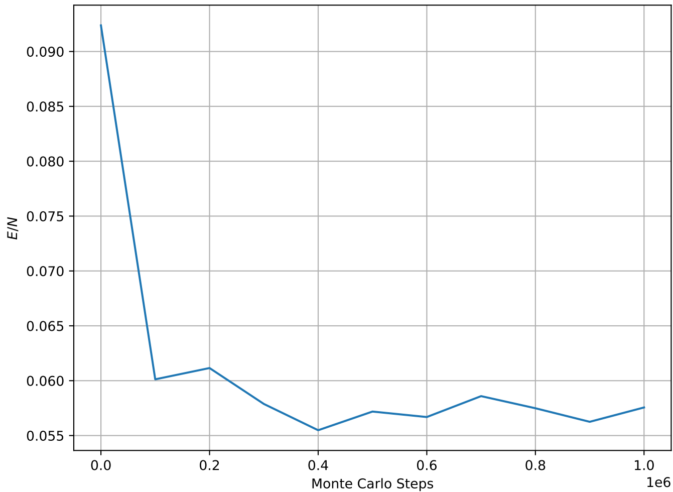
Energy per Spin at T = 6.0e - 02 , L = 64
