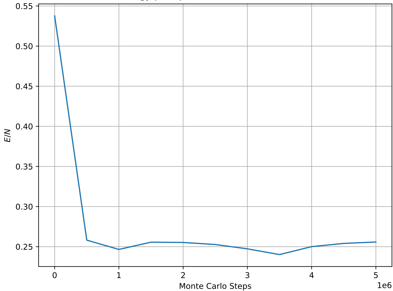
Energy per Spin at T = 1.70e - 01 , L = 32
