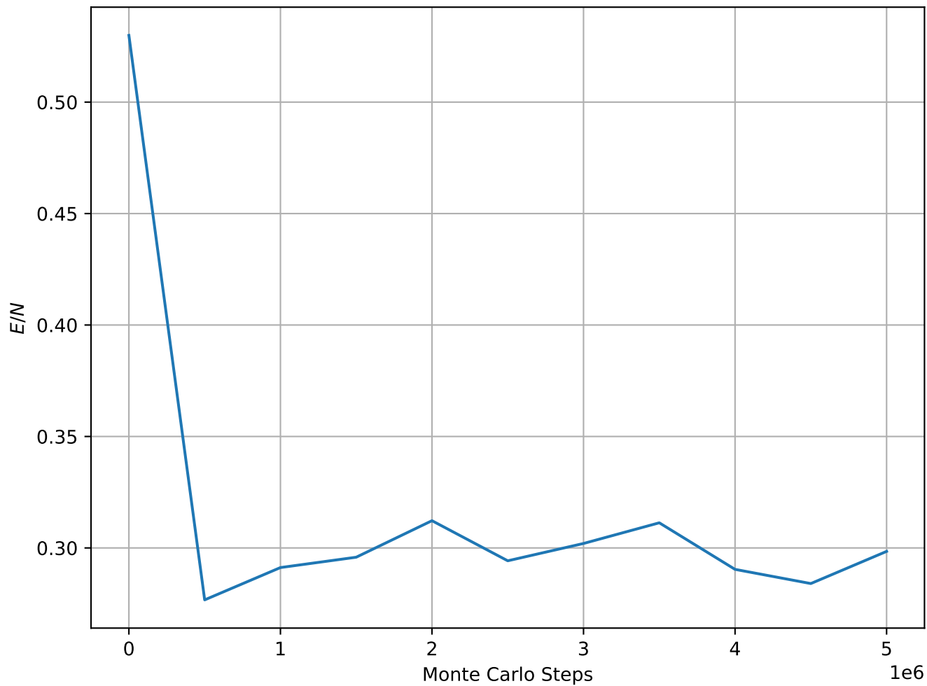
Energy per Spin at T = 1.90e - 01 , L = 32
